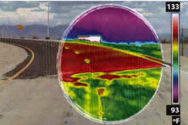
Şekil 7 : Arizona-Mesa’da bir yol kaplamanın temel görüntüsü. Arkadaki asfalt kaplama ile öndeki beton kaplamanın arasındaki sıcak farkı çarpıcıdır.
